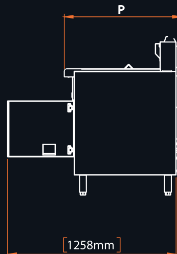
VISÃO LATERAL RBF75
