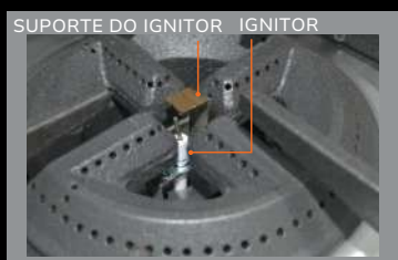
Suporte do ignitor, cujas funções são direcionar e proteger o ignitor
