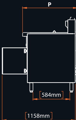
VISÃO LATERAL RBF40/50
